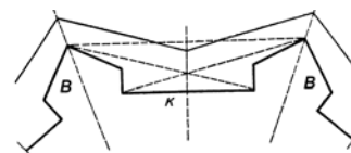
Schemat frontu bastionowego (K – kurtyna, B – bastion).
